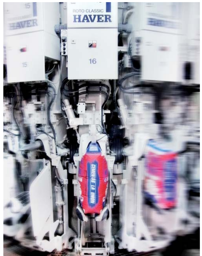
Der Papiersack erlaubt hohe Abfüllgeschwindigkeiten. (Bild: Haver&Boecker)
